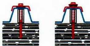
Profil 40/183 Befestigung Dach
